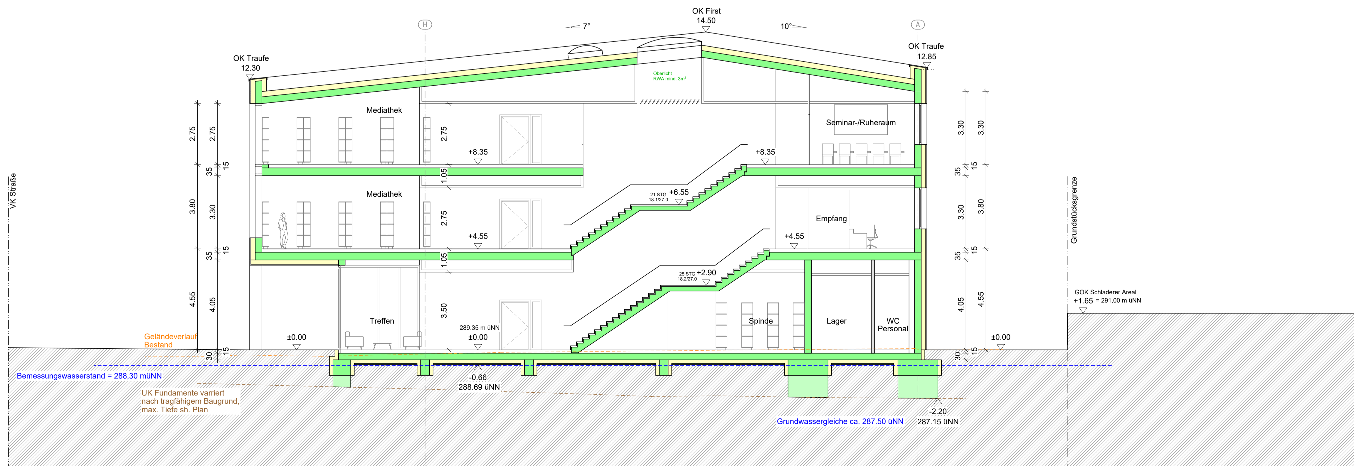
Schnitt B-B
