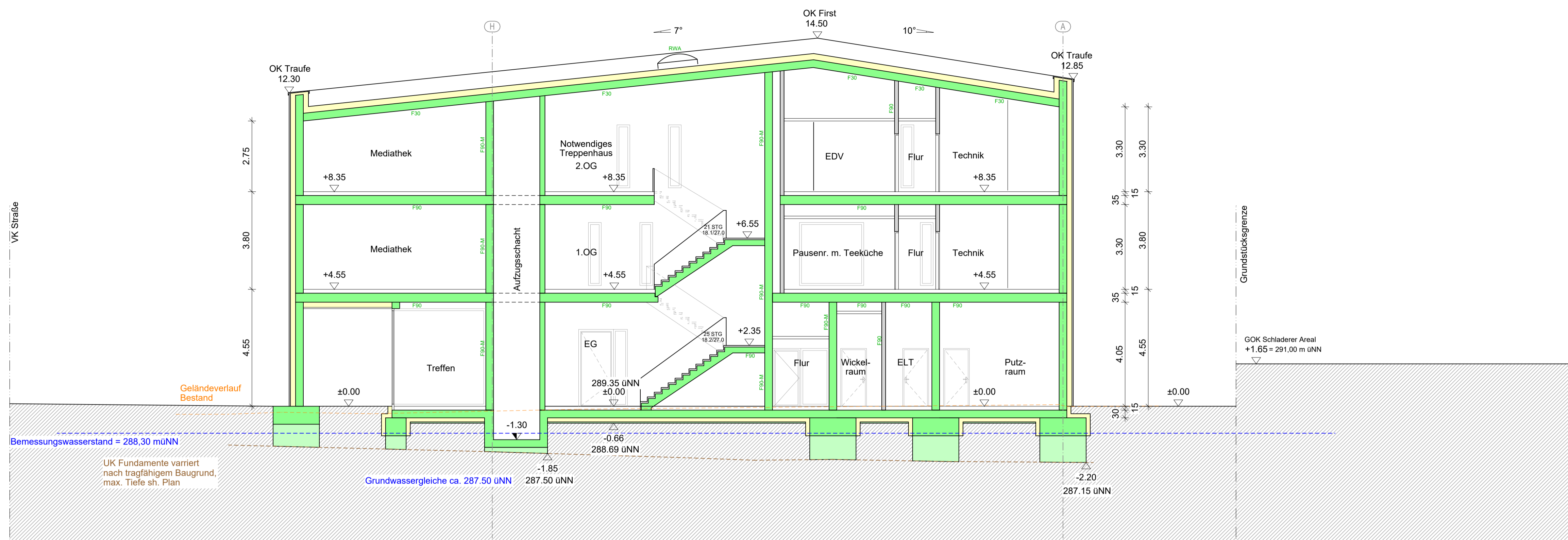
Schnitt A-A
